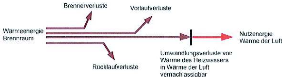
Bild 3.3: Energiefluß der Gasheizung
