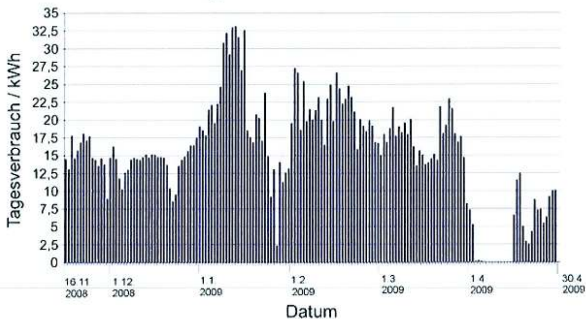
Bild 4.4: Verbrauch der Gruppe 4 (Wohnzimmer)
