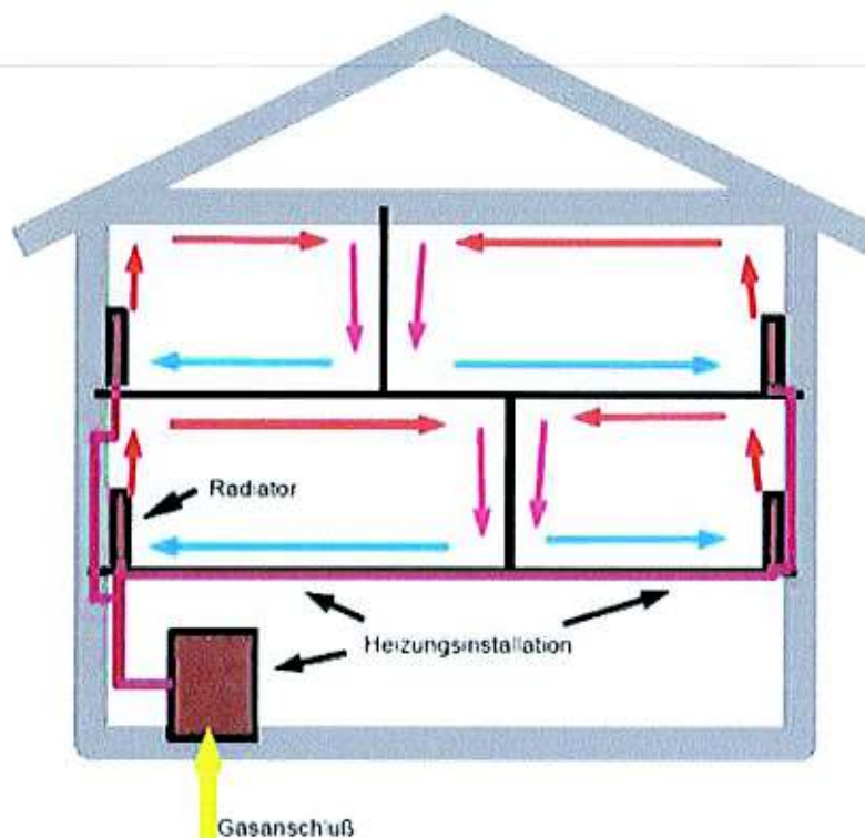
Bild 3.1: Prinzipieller Aufbau einer zentralen Gas-Warmwasserheizung
