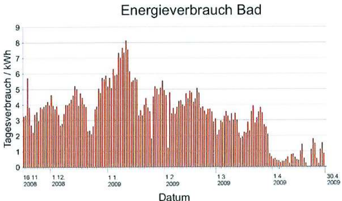
Bild 4.1: Verbrauch der Gruppe 1 (Bad)
