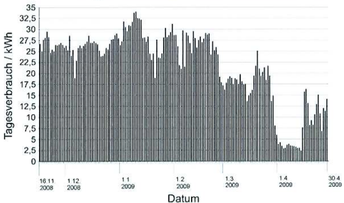
Bild 4.3: Verbrauch der Gruppe 3 (Büro / Schlafzimmer)
