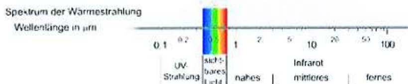
Bild 1.4: Wärmestrahlung im elektromagnetischen Spektrum
