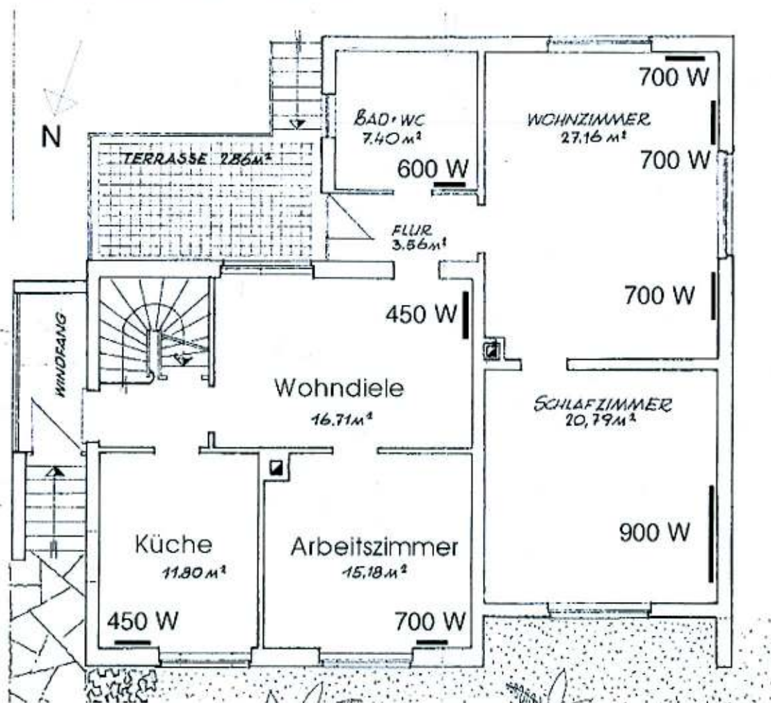
Bild 3.5: Grundriss Erdgeschoss des Maßobjekts
