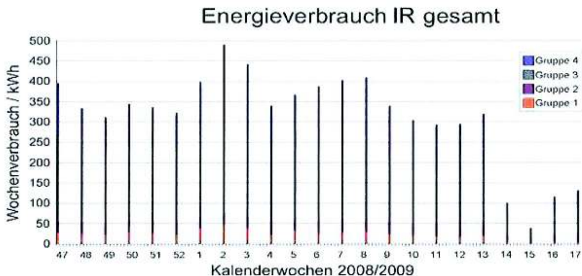
Bild 4.7: Wochen-Energieverbrauch der IR-Heizung
