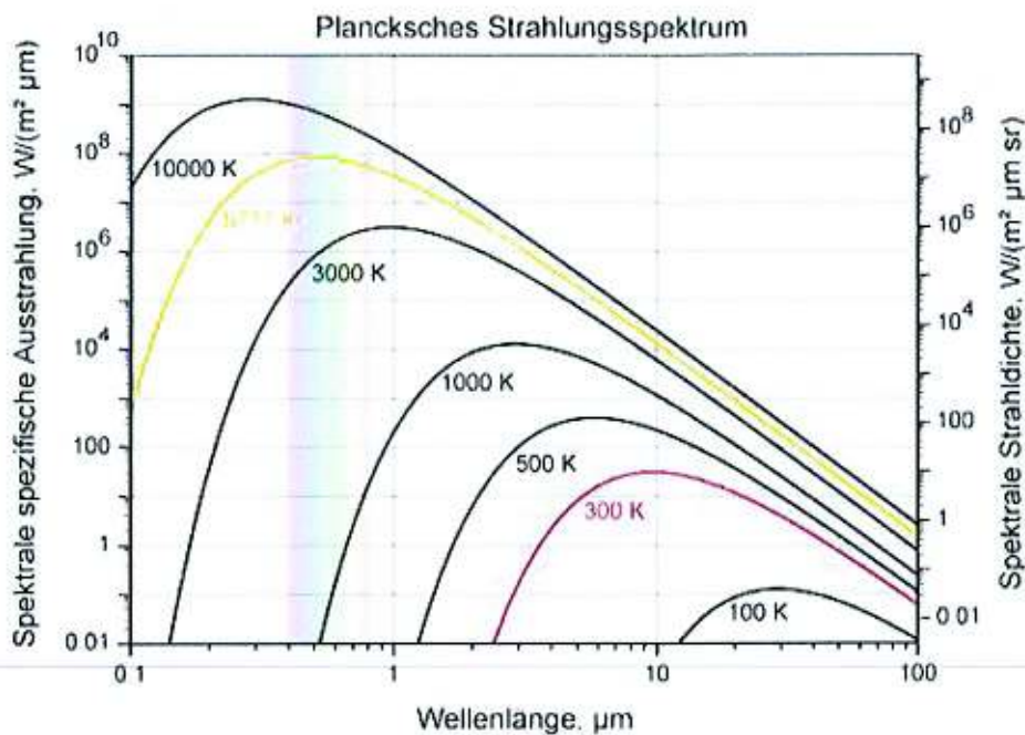
Bild 1.5: Strahlungsspektrum des idealen schwarzen Körpers
