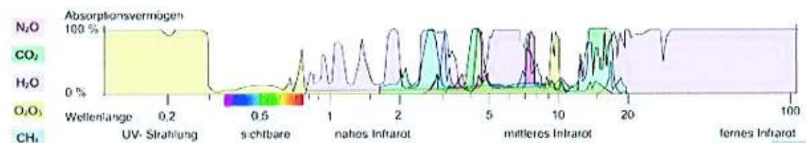
Bild 1.6: Absorptionsspektren verschiedener Stoffe in Luft
