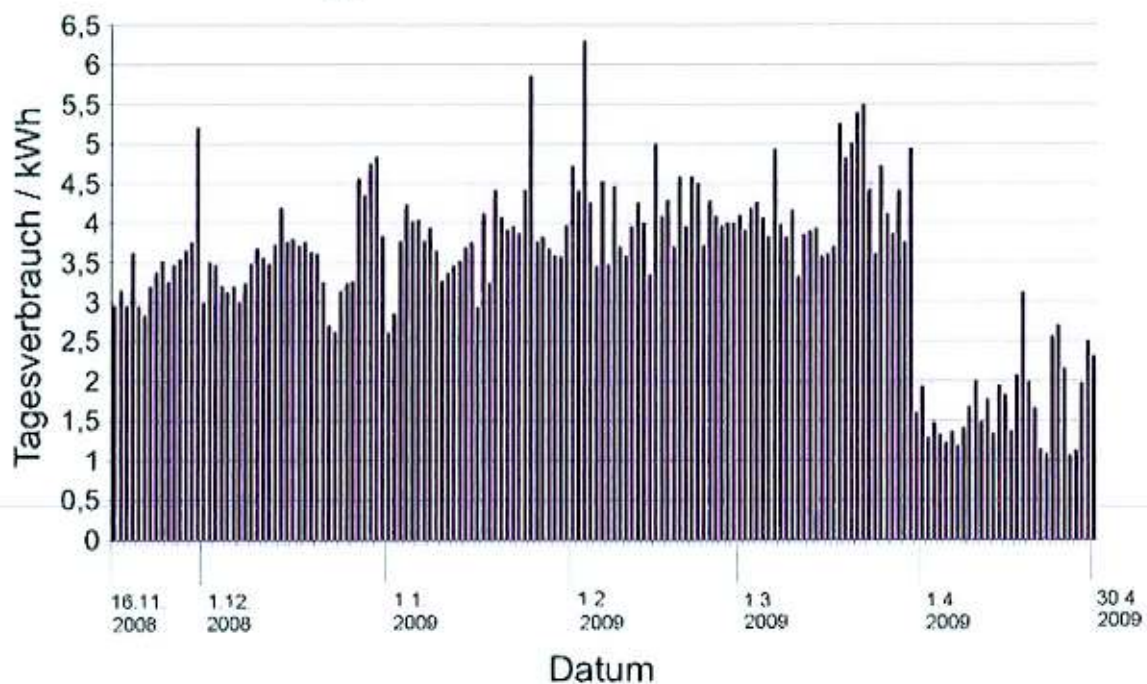
Bild 4.2: Verbrauch der Gruppe 2 (Küche / Wohndiele)
