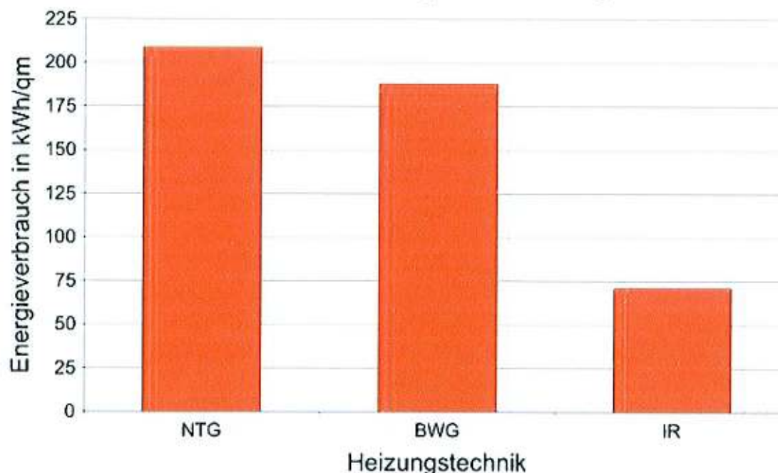
Bild 4.8: Wohnflächenbezogener Energieverbrauch im Vergleich
